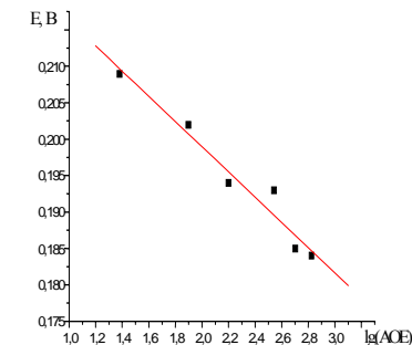
Рис.5 Зависимость окислительно-восстановительного потенциала виноградных вин типа "Кагор" от \lg(\text{AOE}) (Y = (0.233 \pm 0.004) - (0.017 \pm 0.002)\lg X, R = 0.98)
