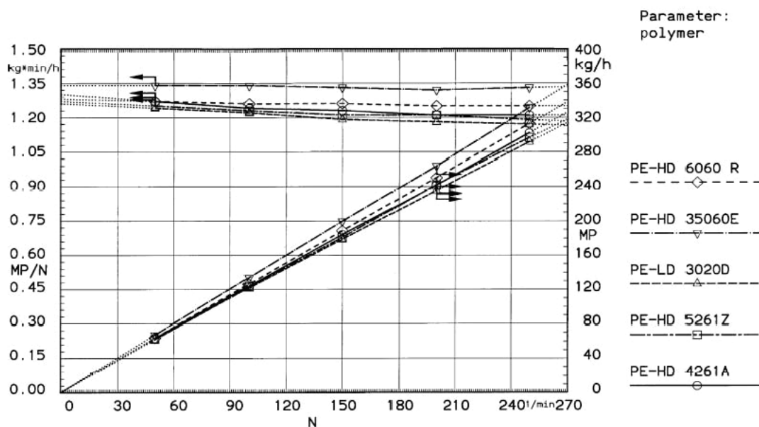
Рис. 3. Расходно-напорная характеристика (линии с большим наклоном) и изменение удельной производительности за оборот (линии с малым наклоном) прессов HELIBAR показывают высокую стабильность работы даже при высоких противодействиях.
